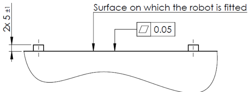
1.2: Montageplatte für Roboterbasis
